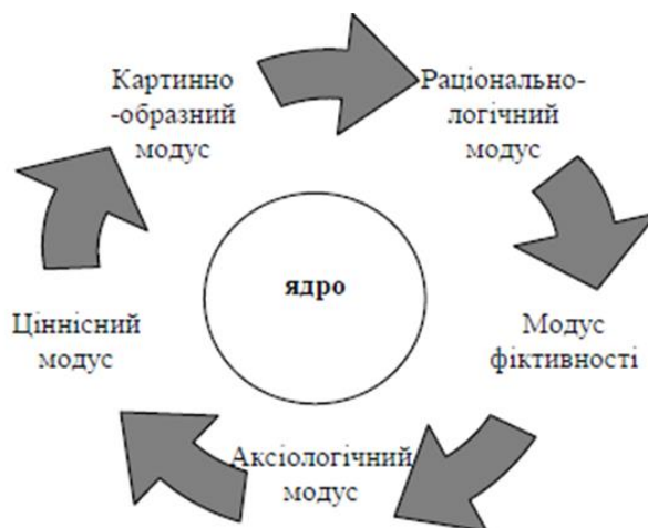
Рис.1 Структура концепту
